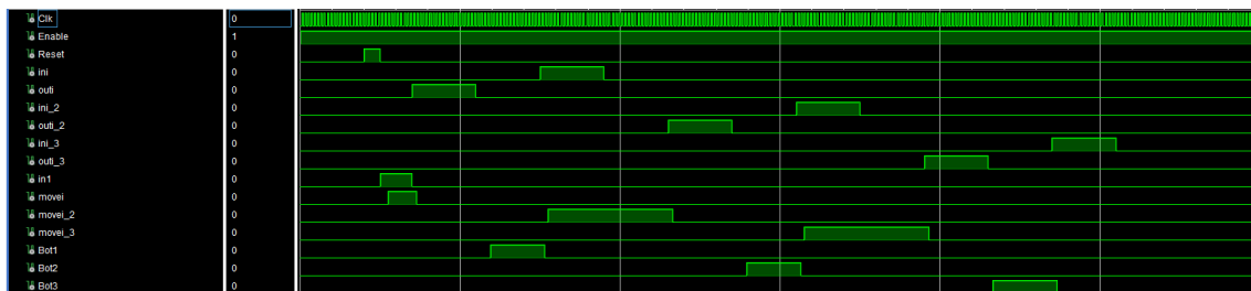
Figura 31: Simulação do sistema distribuído em FPGA com buffers síncronos e atraso entre eventos
