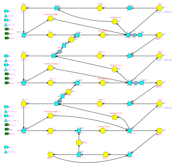
Figura 26: Decomposição do modelo com canais assíncronos
