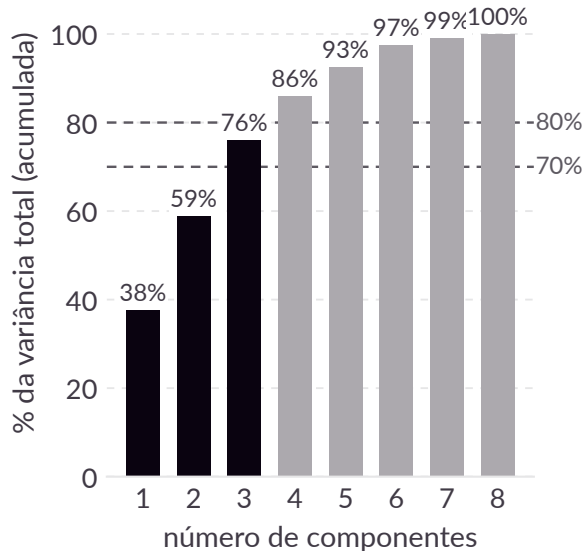
(b) Variância explicada acumulada
