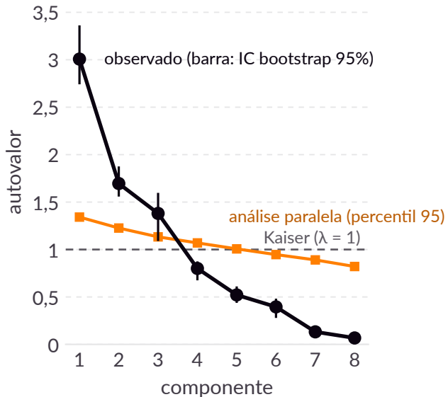
(a) Autovalores de R
