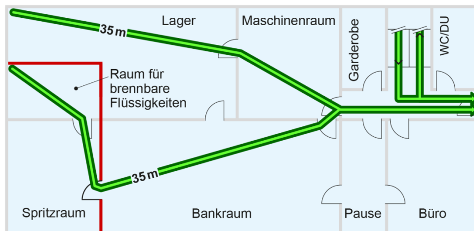
Erdgeschoss
