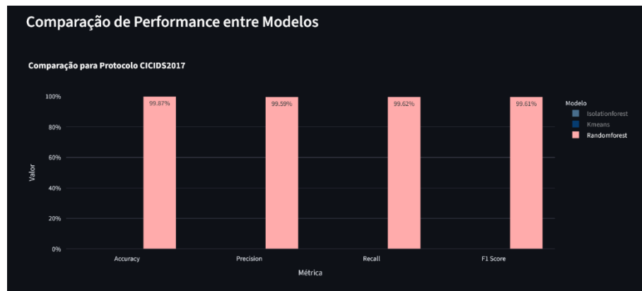
Figura 3.2 – Gráfico de comparação apenas com o Random Forest
