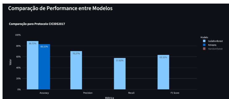
Figura 3.3 – Dashboard de Comparação apenas com o Isolation Forest e K-Means Seleccionados
