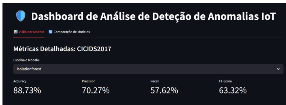
Figura 2 – Dashboard de visualização de métricas do treino de cada modelo
