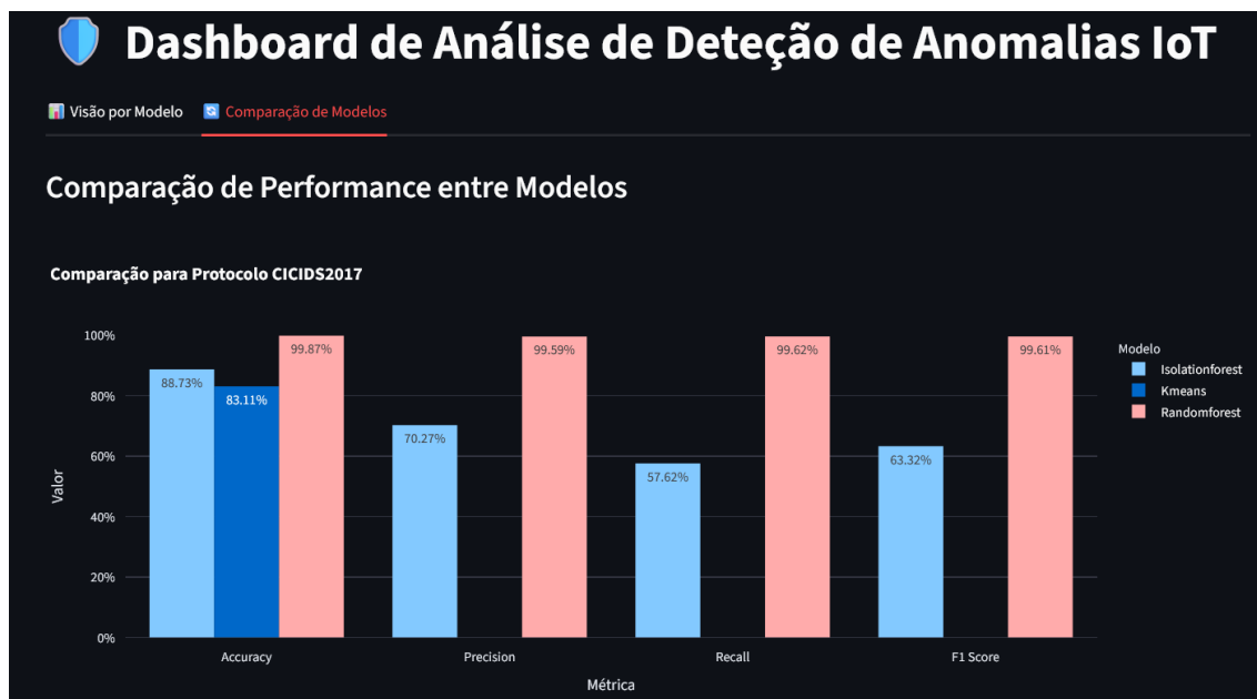
Figura 3.1 – Dashboard de comparação de modelos
