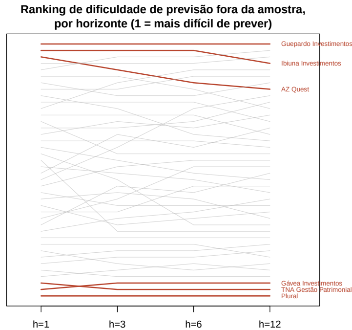
Figura 6: Estabilidade do ranking de dificuldade por gestora entre os quatro horizontes, em 40 gestoras com dado completo.
