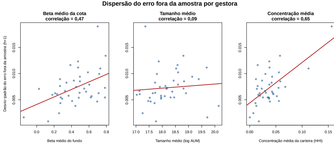
Figura 5: Desvio-padrão do erro fora da amostra por gestora contra o beta médio, o tamanho médio e a concentração média da carteira, em 40 gestoras.
