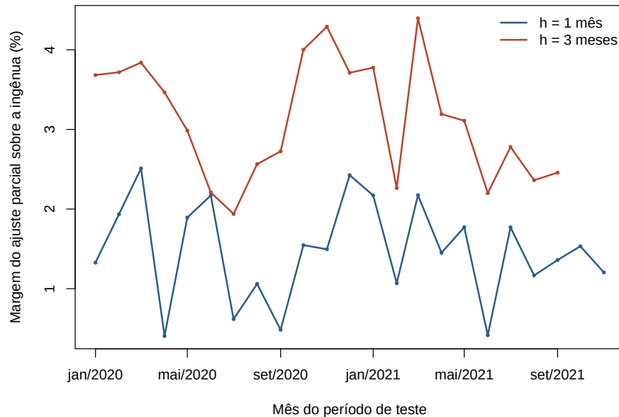
Figura 1: Margem do ajuste parcial sobre a previsão ingênua, mês a mês, no período de teste.
