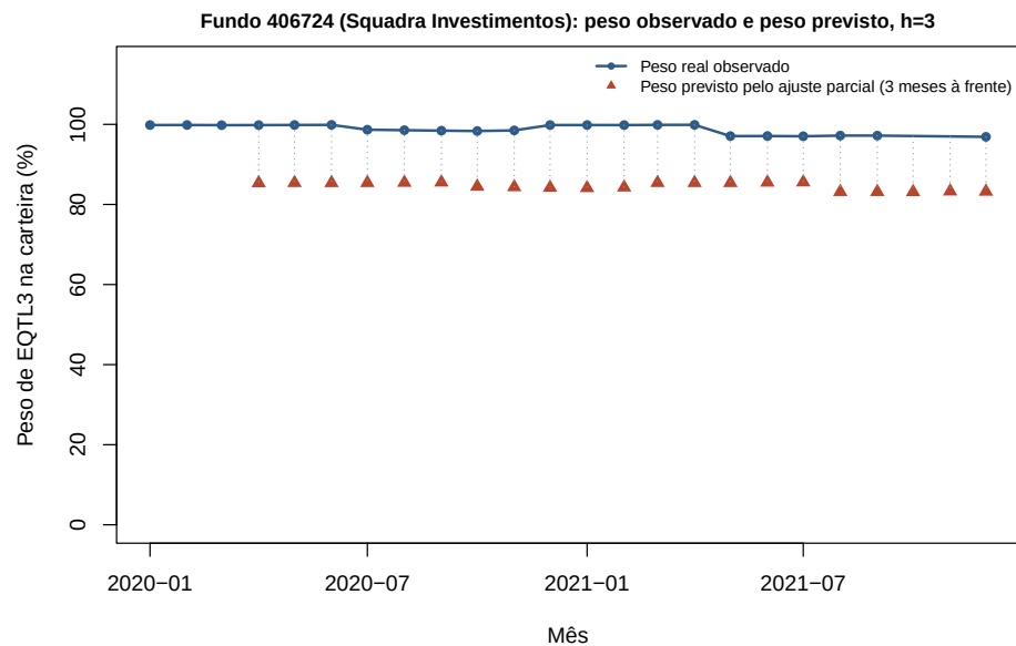
Figura 3: Peso observado e peso previsto no horizonte de três meses para o par de fundo e ativo de maior erro fora da amostra entre os que mantêm posição relevante.
