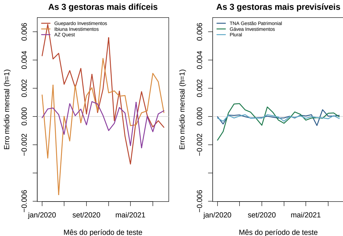
Figura 2: Evolução mensal do erro médio fora da amostra no horizonte de um mês, para as três gestoras de maior e as três de menor erro.
