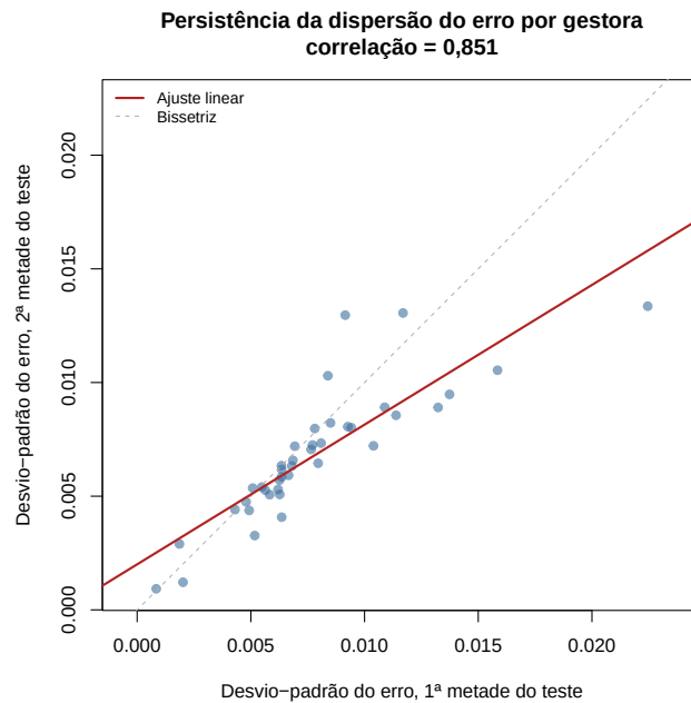
Figura 4: Desvio-padrão do erro fora da amostra na primeira metade do período de teste, em 2020, contra a segunda metade, em 2021, por gestora. A linha tracejada é a bissetriz.
