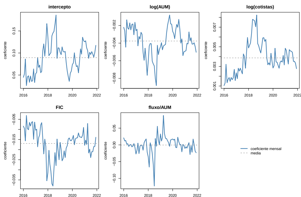
Figura 1: Coeficientes da regressão mês a mês, de 2016 a 2021. A linha tracejada marca a média de cada série.
