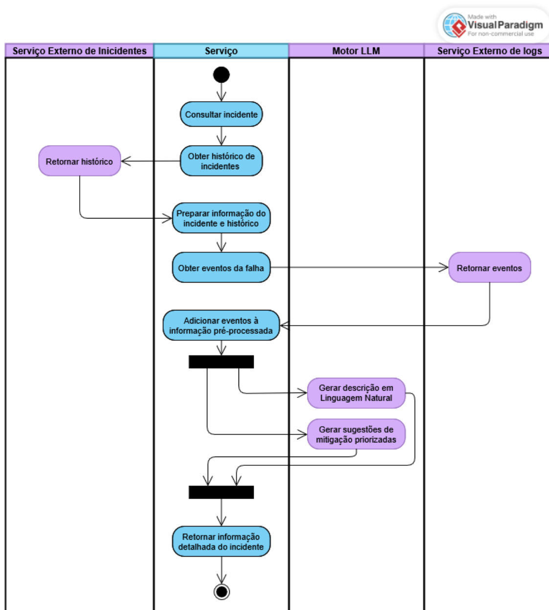
Figura 3.2: Diagrama de Atividade
