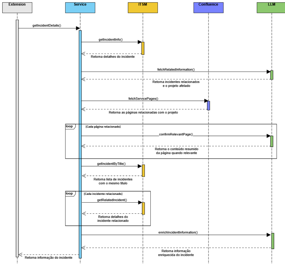
Figura 4.8: Diagrama de Sequência
