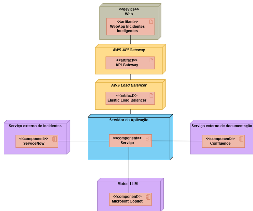
Figura 4.7: Diagrama de Implantação
