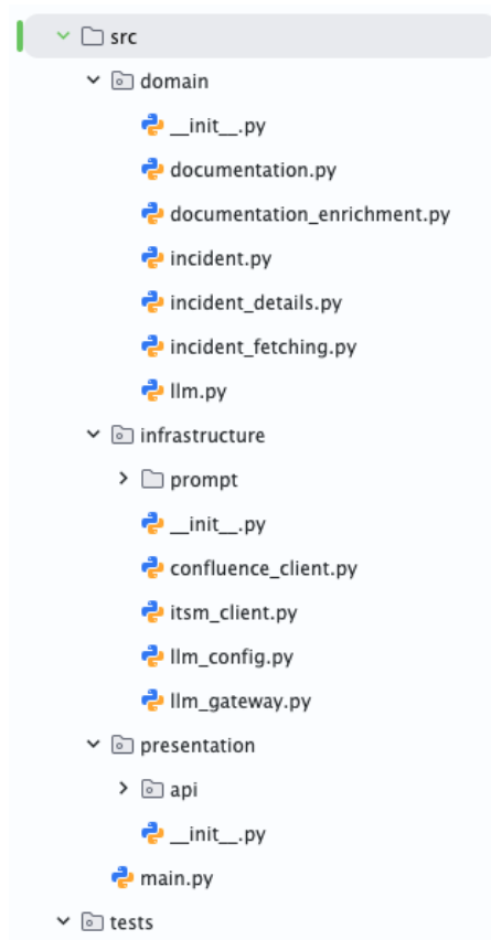
Figura 5.2: Estrutura do Protótipo
