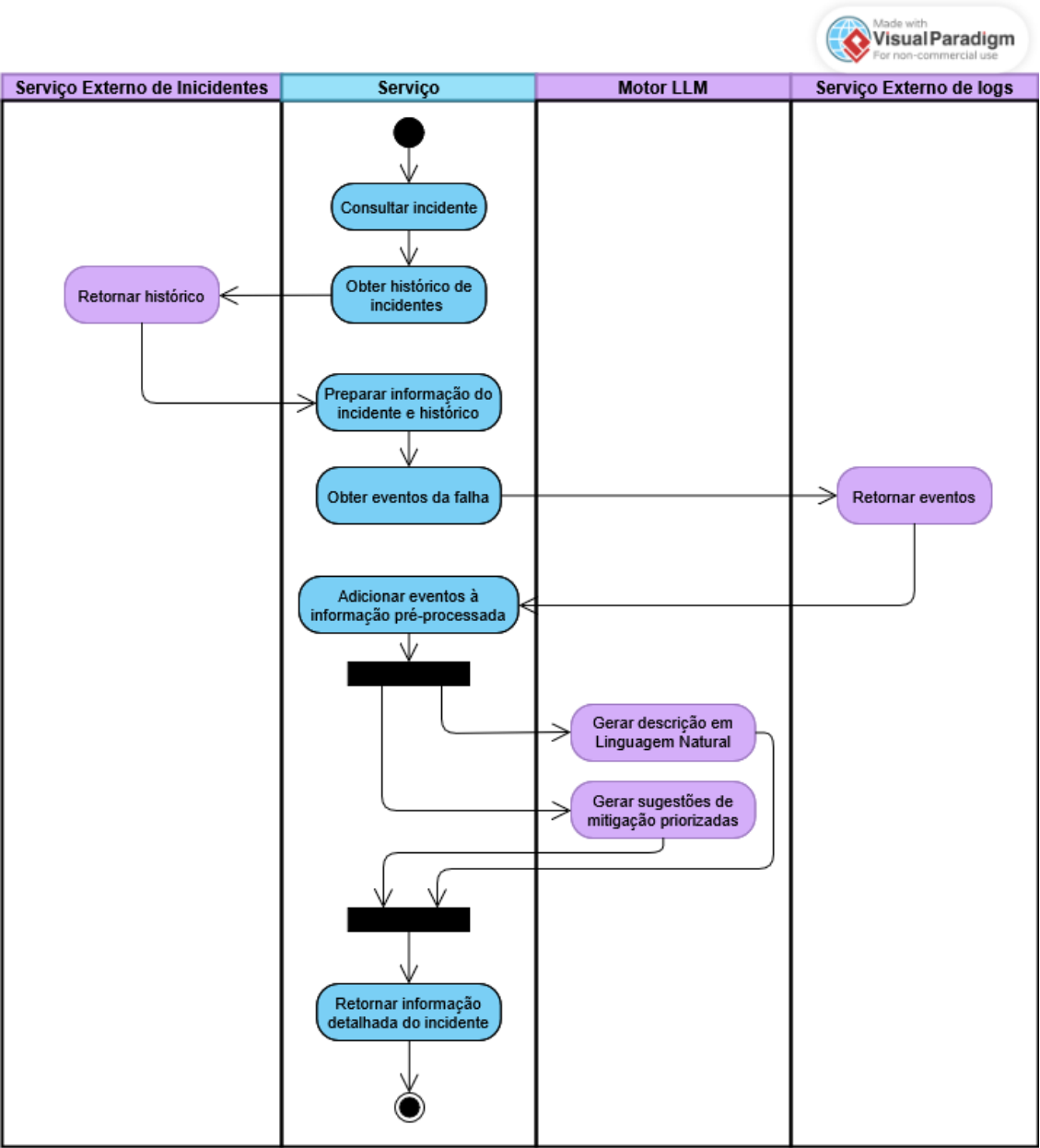
Figura 3.2: Diagrama de Atividade
