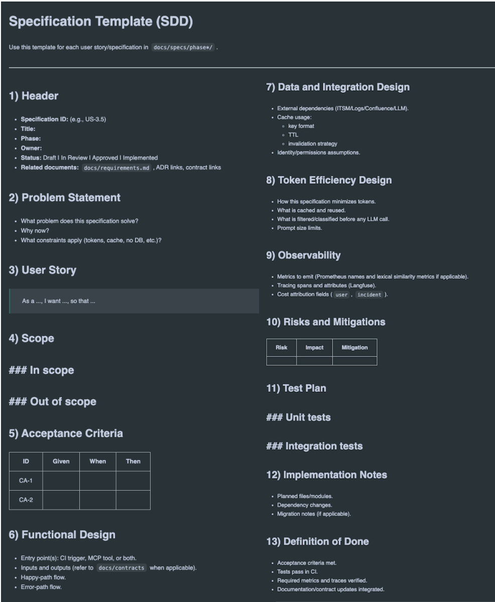
Figura 6.1: Modelo Base de uma Especificação
