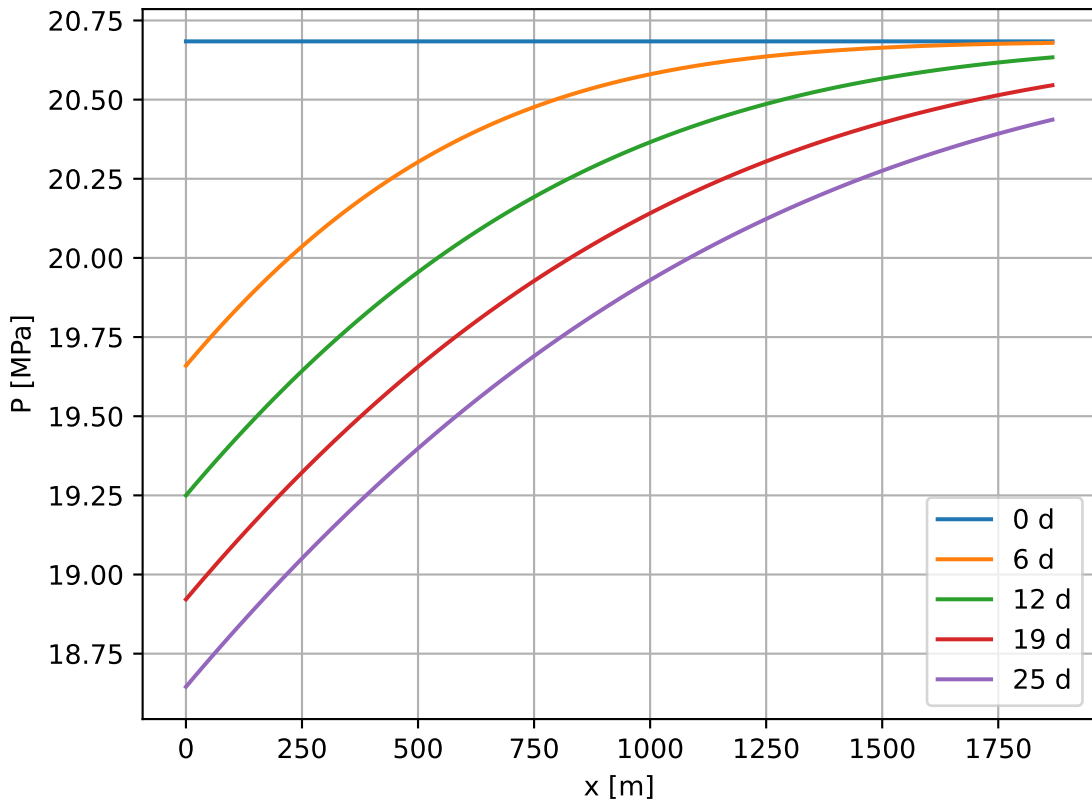
Fluxo linear transiente - Condição de Fluxo-Pressão
