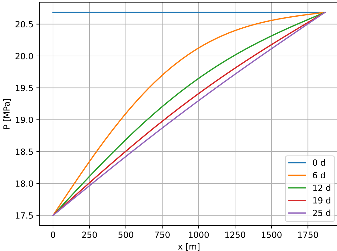
Fluxo linear transiente - Condição de Pressão-Pressão
