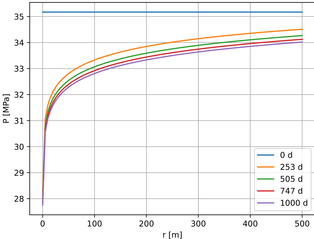
Fluxo radial transiente - Condição de Fluxo-Pressão
