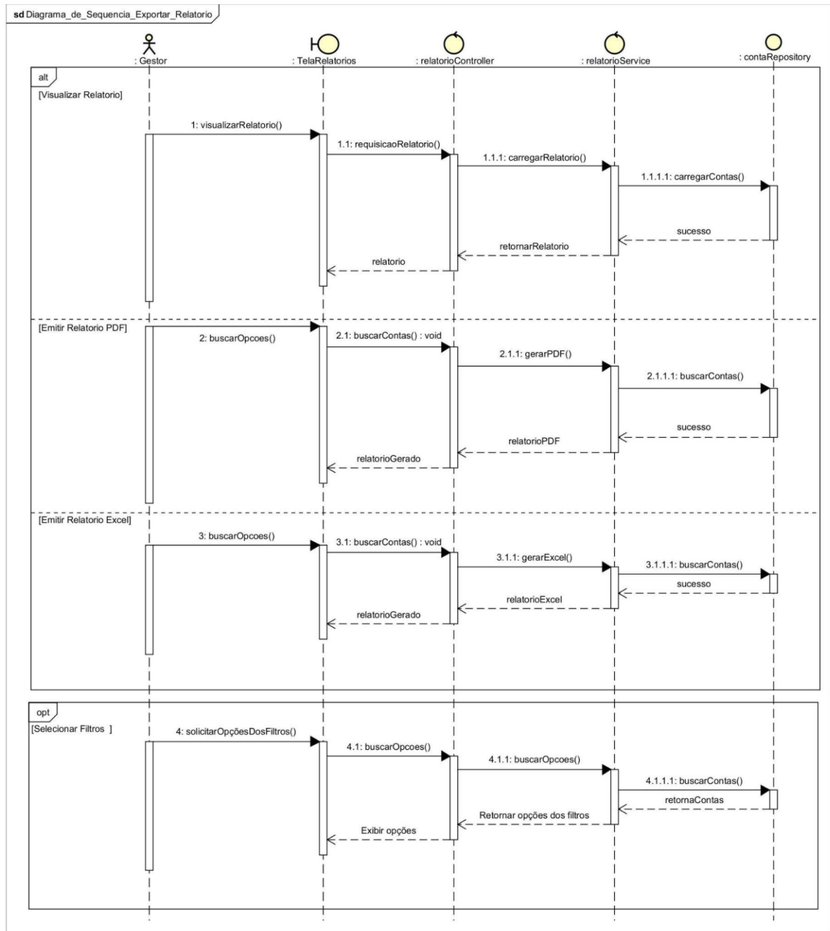
Figura 8 – Diagrama de Sequência - Exportar Relatório
