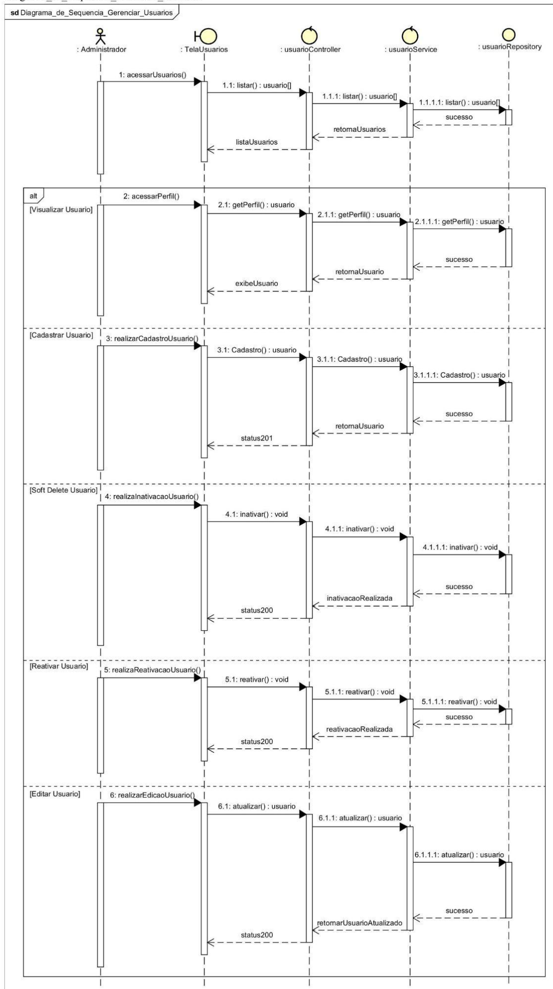
Diagrama de Sequencia Gerenciar Usuarios
