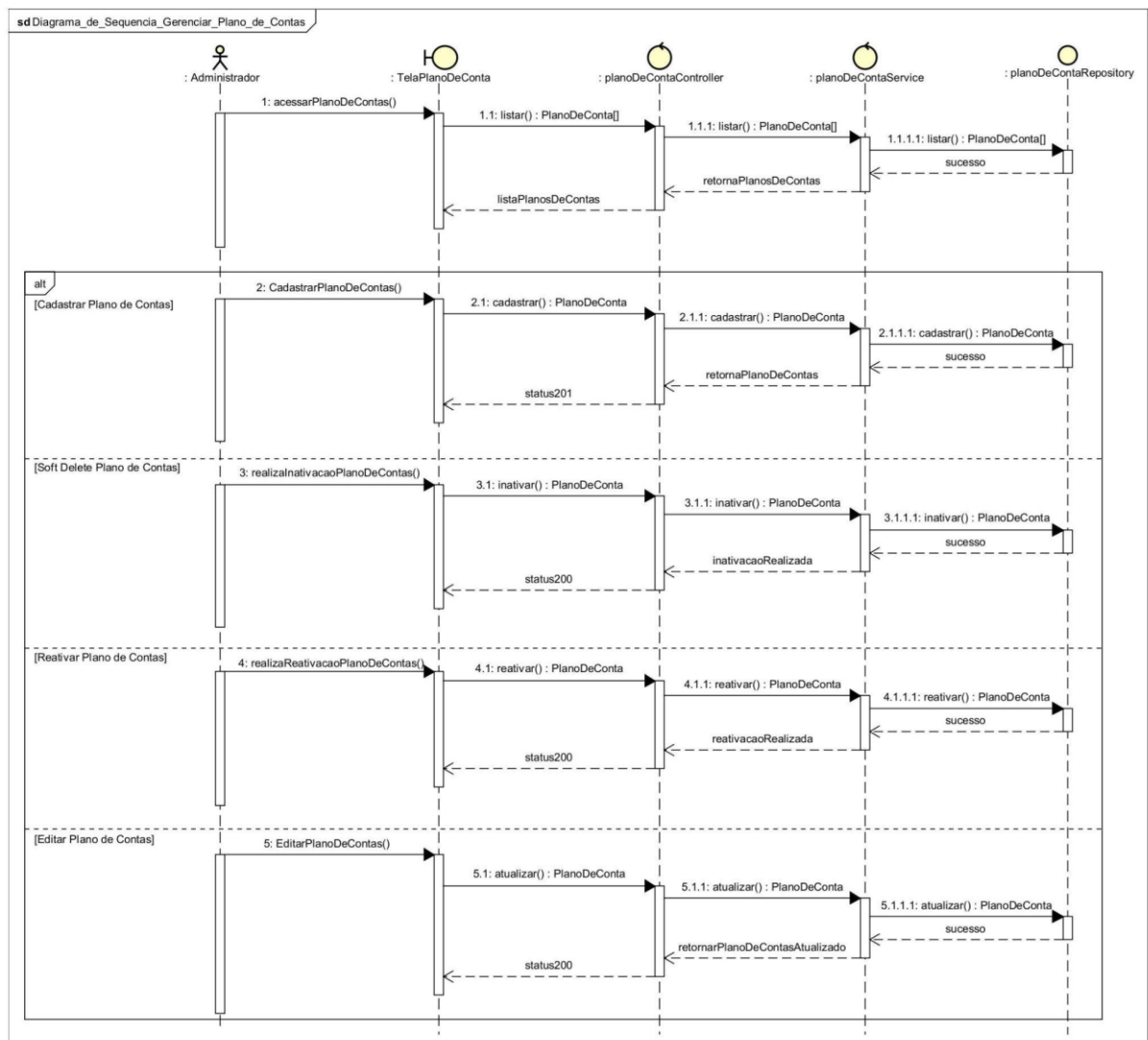
Figura 7 – Diagrama de Sequência - Gerenciar Plano de Contas
