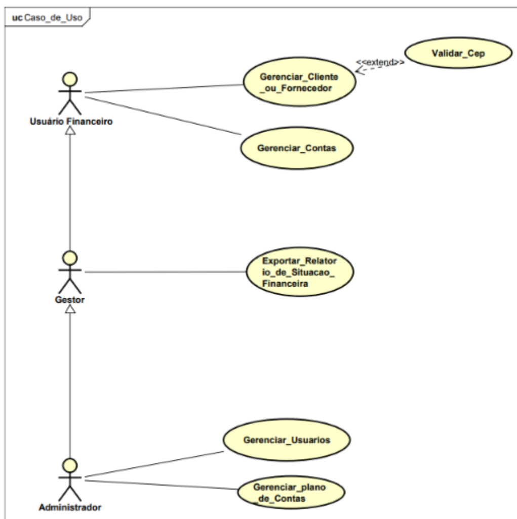
Figura 1 – Diagrama Caso de Uso
