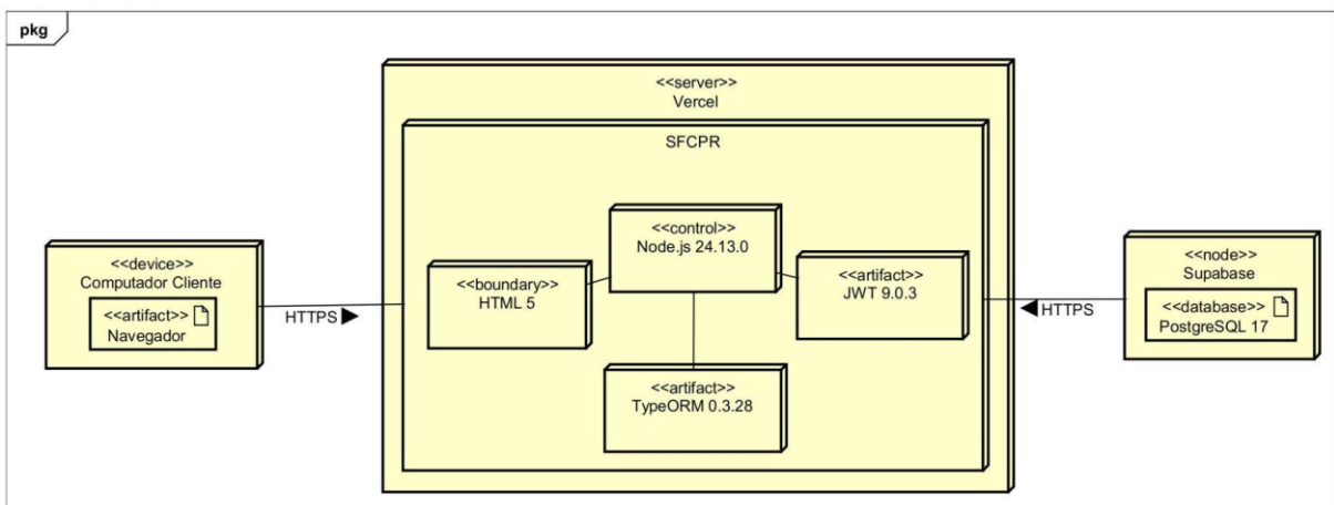
Figura 10 – Diagrama de Implantação
