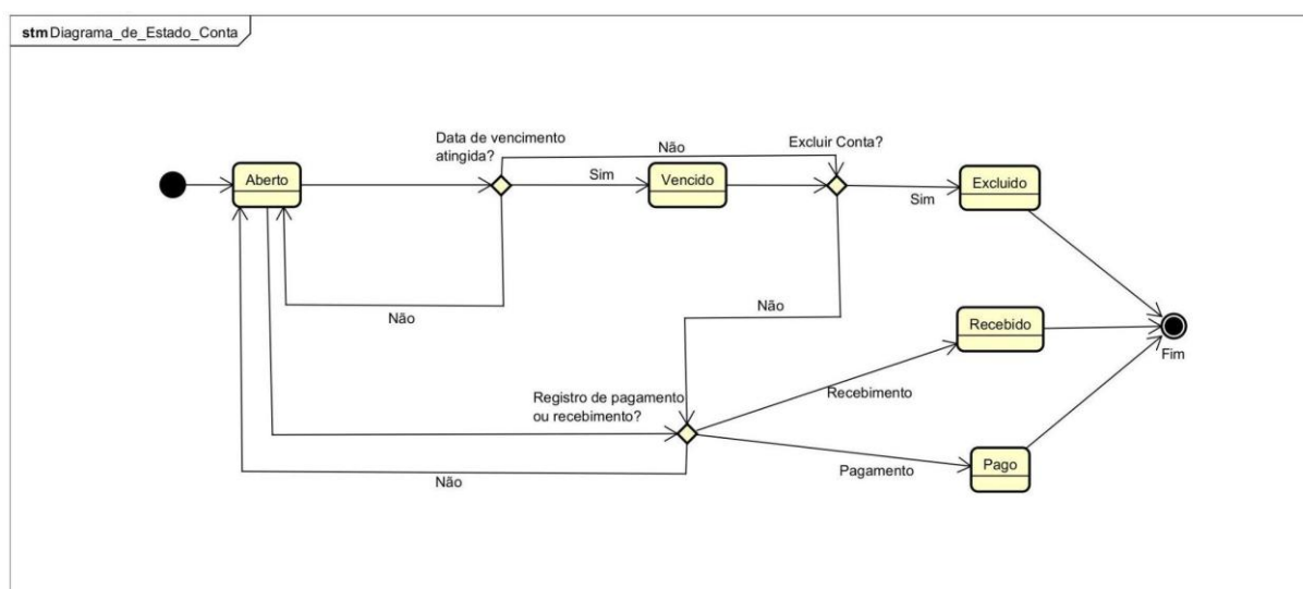
Figura 9 - Diagrama de Estado - Conta Financeira
