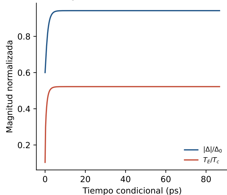
Recuperación en una celda BCS
