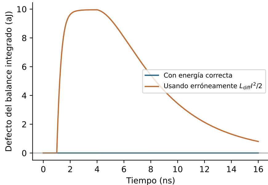
Energía: integrar I d\Phi_{\text{ext}}
