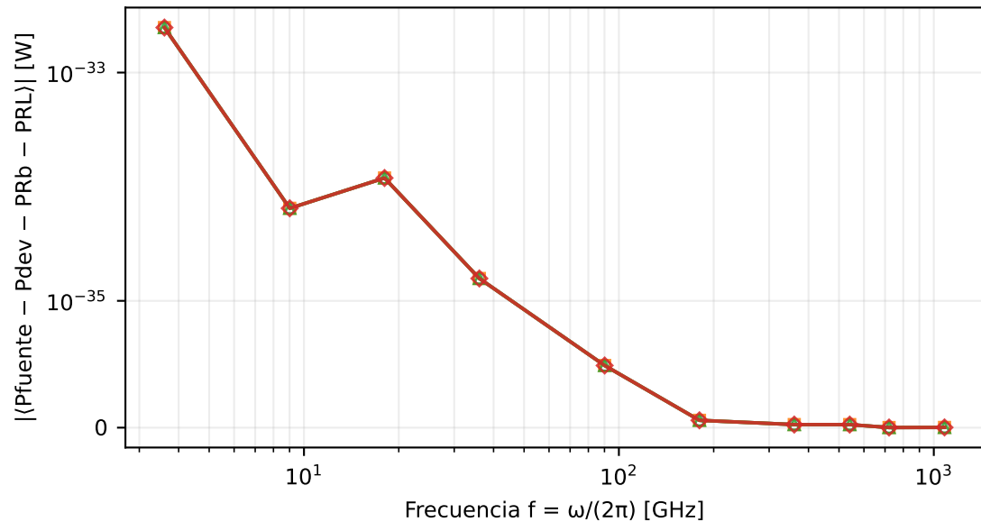
Balance medio del circuito de tres estados
