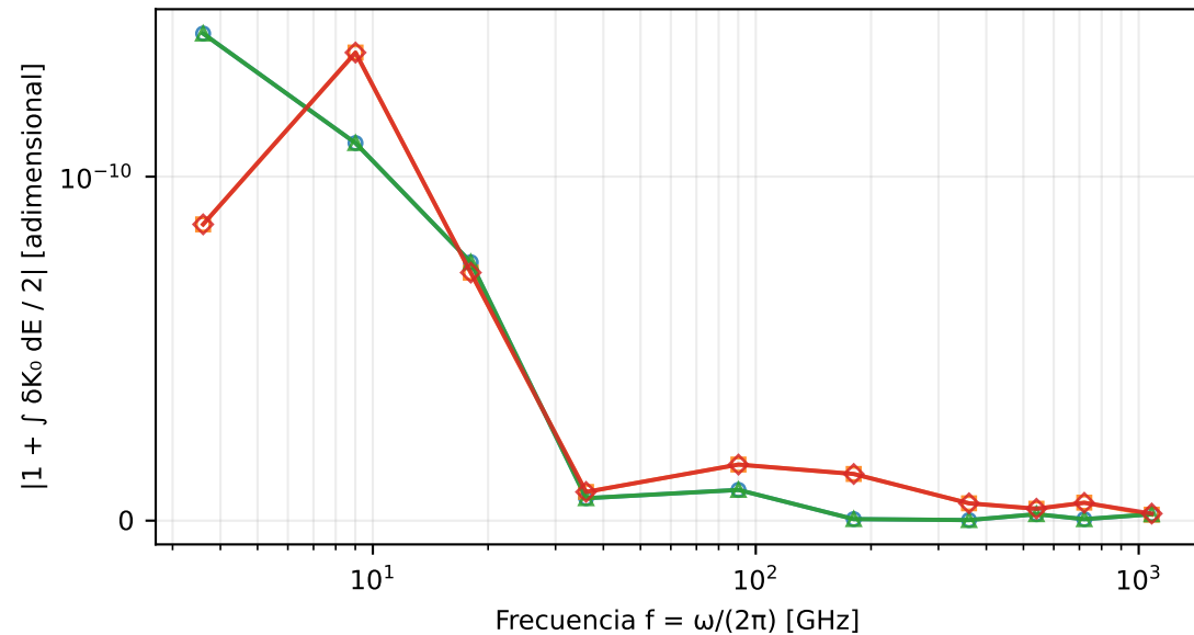
Residuo de calibre: integral con colas resueltas
