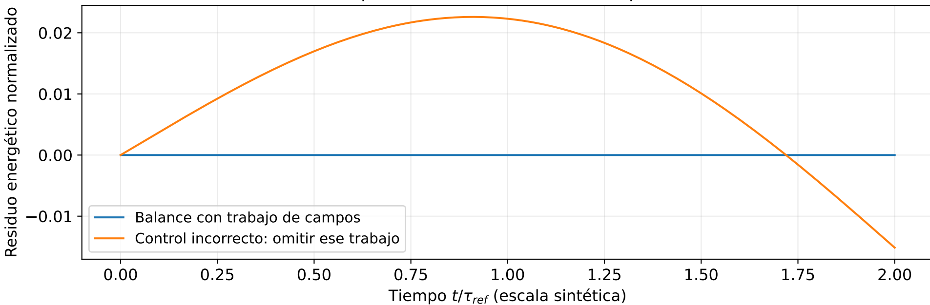
Espectro móvil: la contabilidad importa
