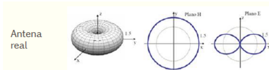
Figura 33: Antena real
