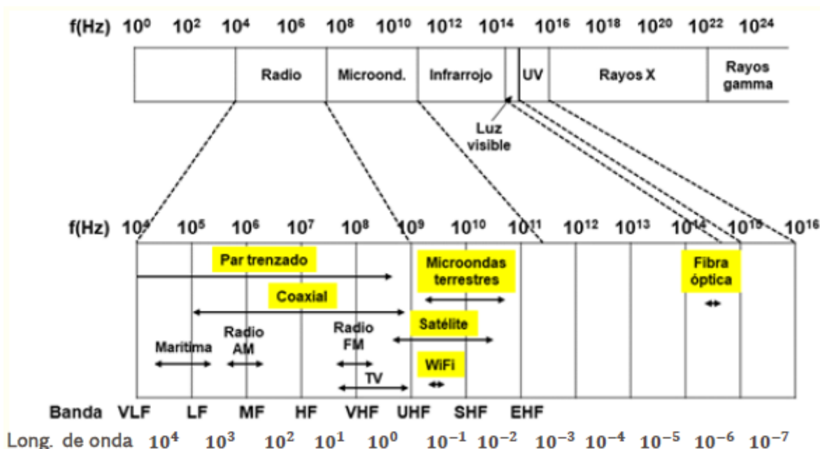
Figura 25: Espectro electromagnetico
