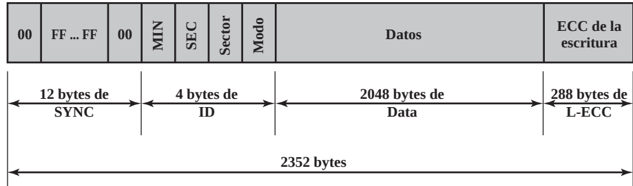
Figura 6.12. Formato de los bloques de un CD-ROM.
