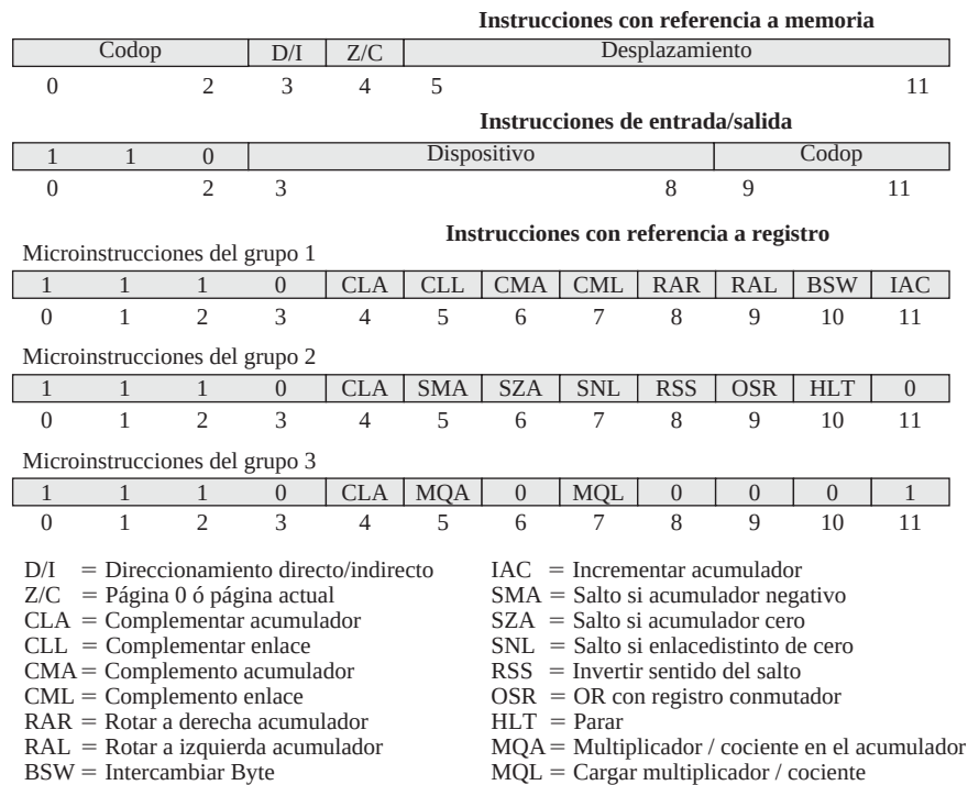
Figura 11.4. Formatos de instrucciones del PDP-8.
