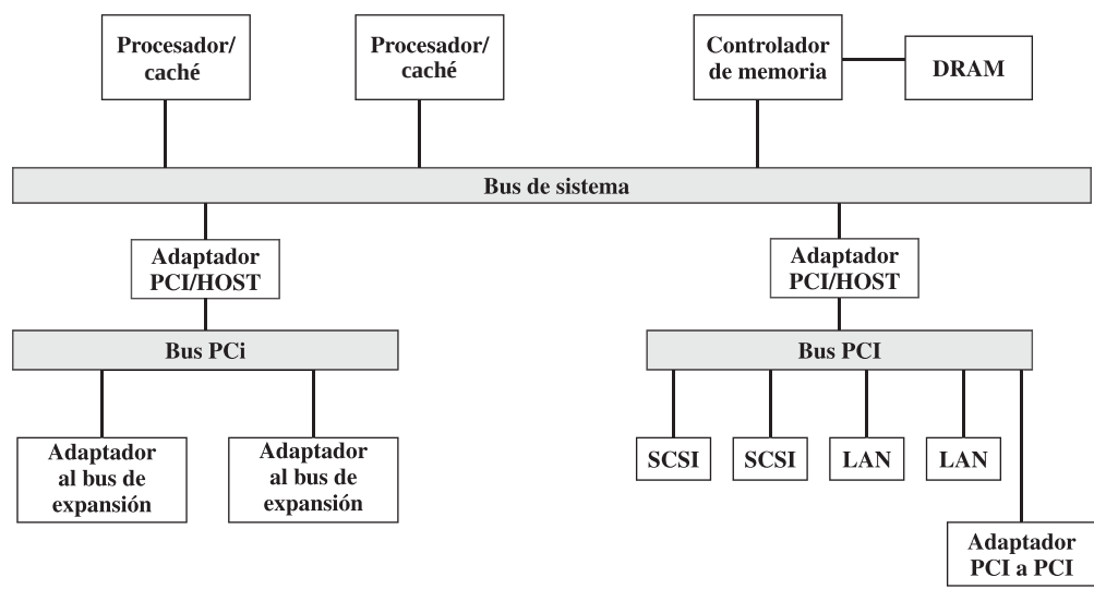
(b) Servidor típico
