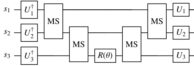
Figura 2: Compilación de e^{-i\theta V} para un generador de soporte w = 3 que factoriza (modelo del Apéndice B del paper): diagonalización local, escalera de 2(w-1) = 4 compuertas MS con una rotación parametrizada al centro, y deshacer la diagonalización.
