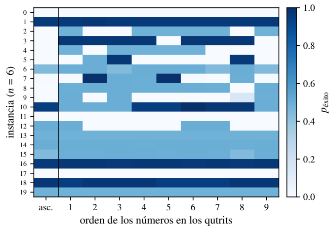
Figura 8: p_{\text{éxito}} de las 20 instancias de n=6 ( \ell=1 , warm) bajo 10 órdenes. La primera columna es el orden ascendente.
