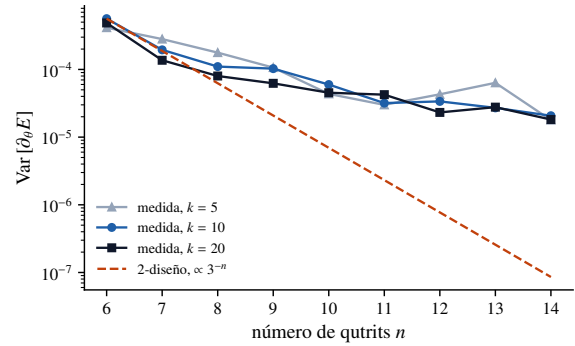
Figura 10: Varianza del gradiente en puntos aleatorios contra n , con la referencia de un 2-diseño anclada en n = 6 .
