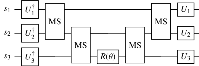
Figura 2: Compilación de e^{-i\theta V} para un generador de soporte w = 3 que factoriza (modelo del Apéndice B del paper): diagonalización local, escalera de 2(w-1) = 4 compuertas MS con una rotación parametrizada al centro, y deshacer la diagonalización.
