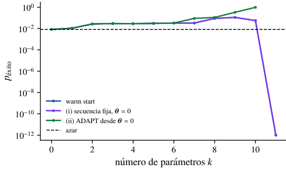
Figura 9: p_{\text{éxito}} contra número de parámetros, n = 6 , una instancia, \ell = 1 . Warm llega a 0.11 y la pierde; ADAPT desde \theta = 0 termina en 0.97.
