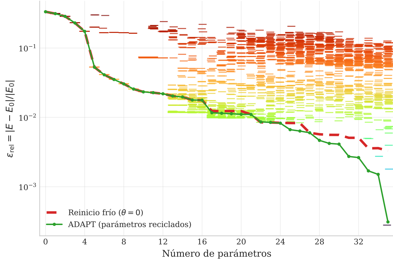
Grafo completo K_6 (15 aristas), \ell = 2 18/35 parámetros
