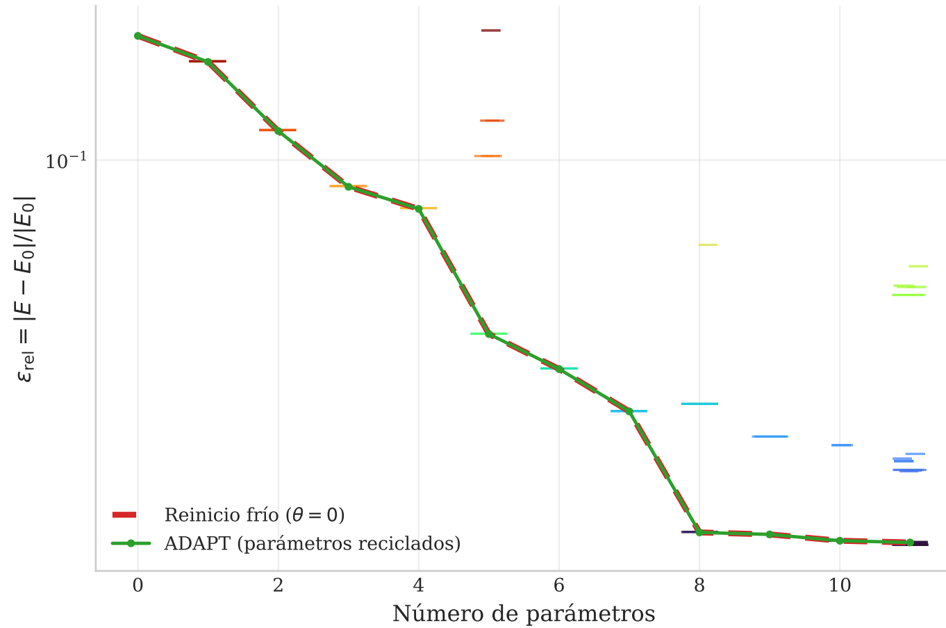
Grafo completo K_6 (15 aristas), \ell = 1 11/35 parámetros (parcial)
