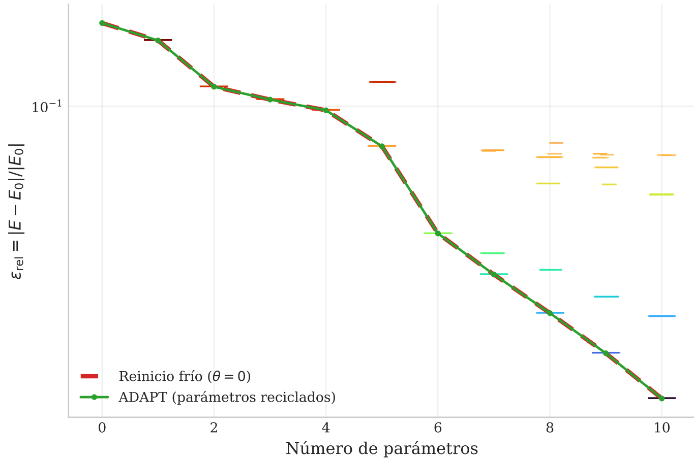
Grafo completo K_6 (15 aristas), \ell = 2 10/35 parámetros (parcial)
