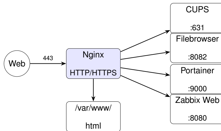
FIGURA 8: Arquitectura del servidor web: Nginx como proxy inverso y servidor de contenido en Debian
