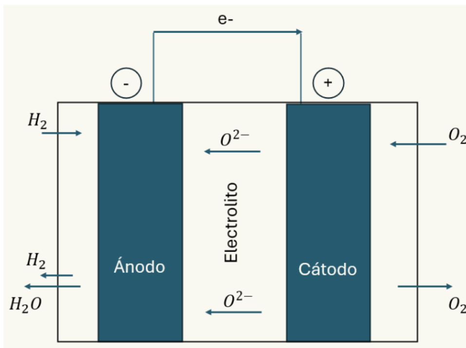
Figura 2. Funcionamiento SOFC, basado en [3]
