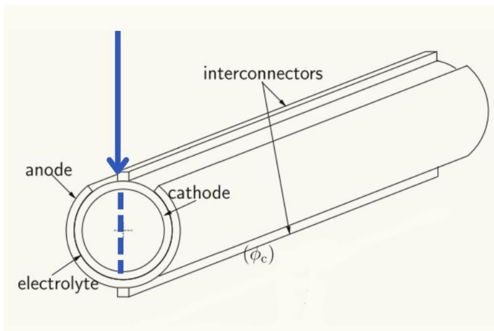
Figura 1. SOFC tubular [2].
