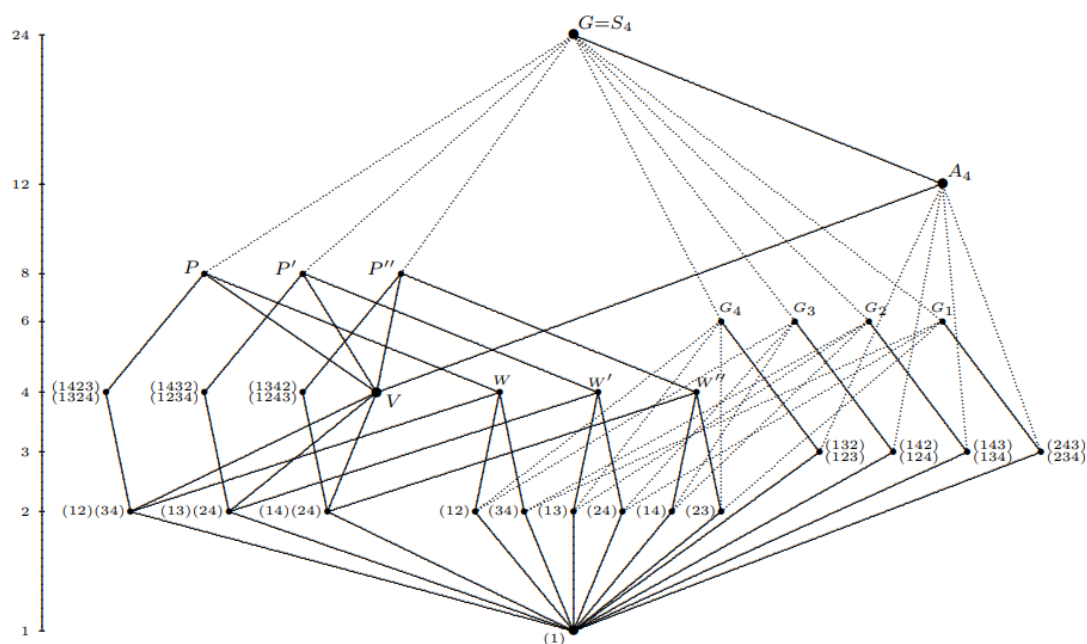
Figure 9.1: Der Verband der Untergruppen der Gruppe S_4 ; vgl. Abb. 3.1 Mit freundlicher Genehmigung von C.M. Ringel
