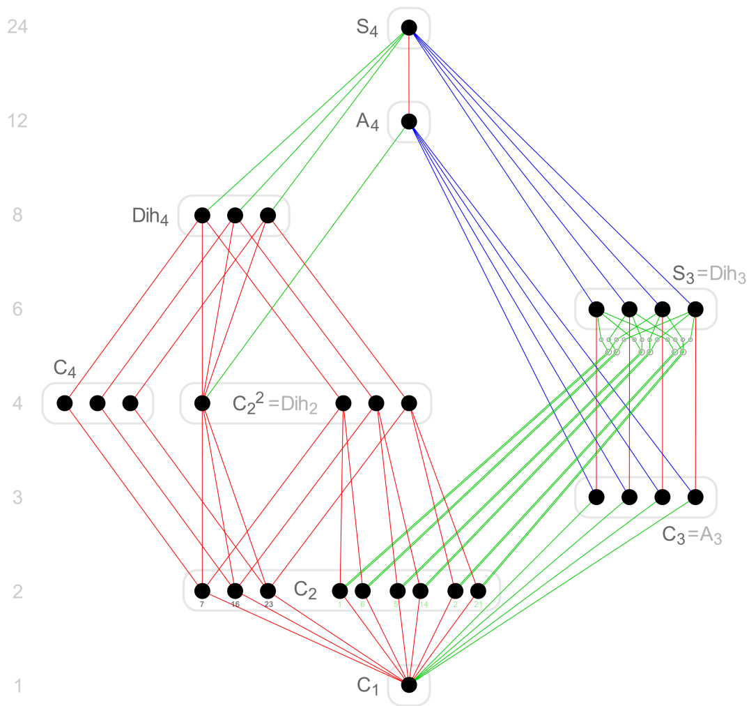
Figure 3.1: Der Verband der Untergruppen der Gruppe S_4
