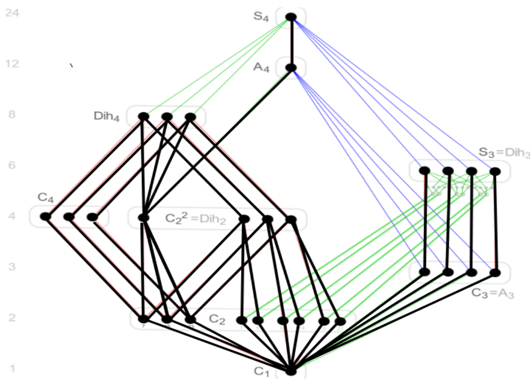
Figure 9.1: Normalteiler in der Gruppe S_4 ; vgl. Abb. 3.1 “dicke” Linien bedeuten “Normalteiler” zwischen den jeweiligen Endpunkten
