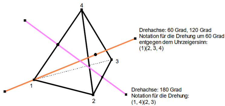
Figure 2.2: Räumliche Drehungen eines Tetraeders
