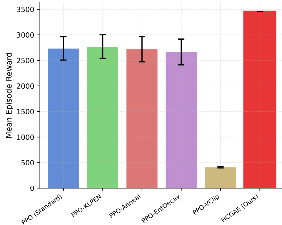
Hopper-v4
