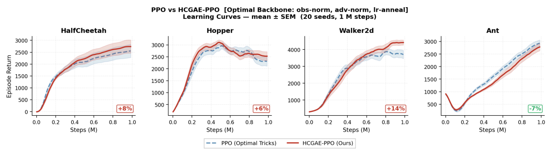
图 1: PPO 学习曲线 (Optimal Backbone)
