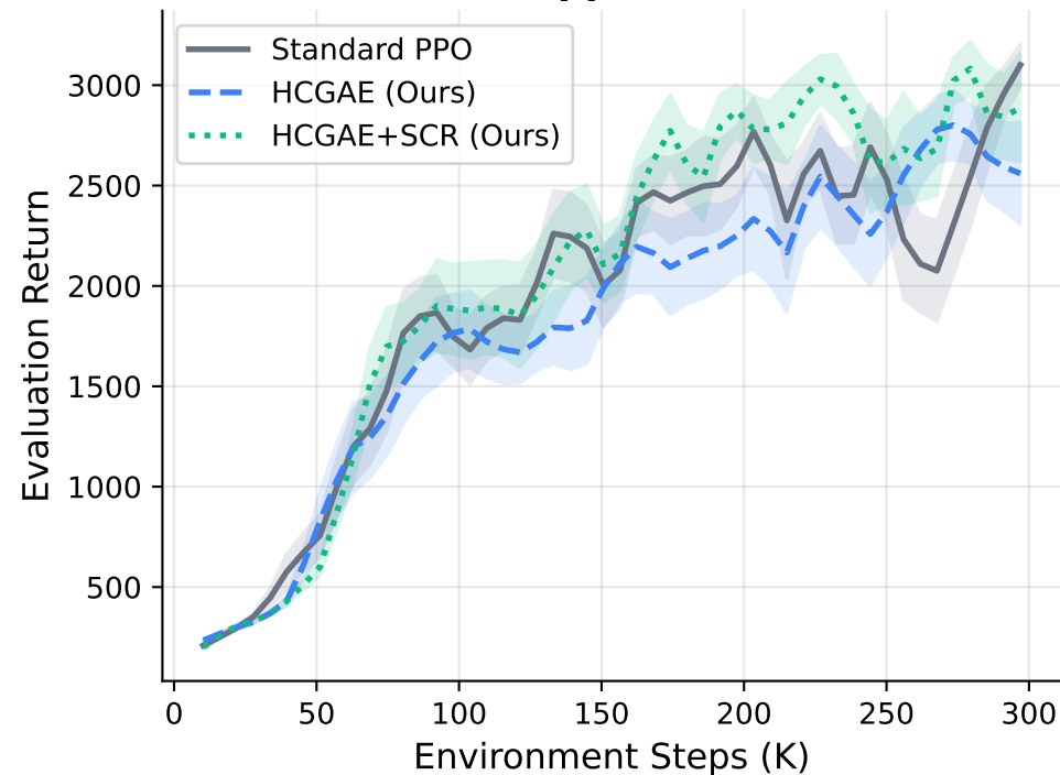
Hopper-v4
