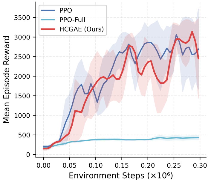
Hopper-v4
