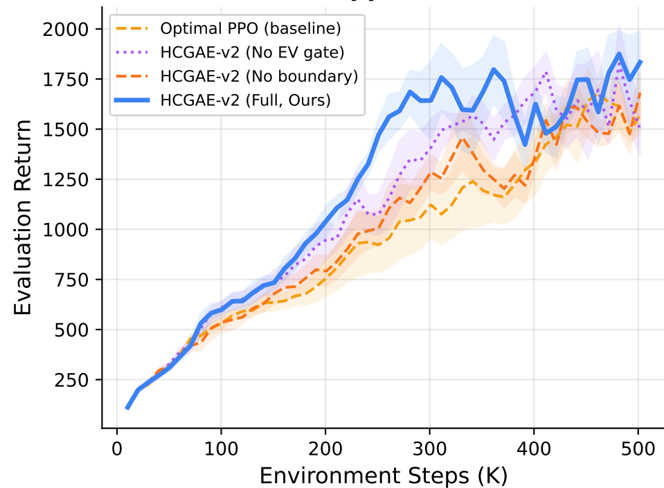
Hopper-v4
