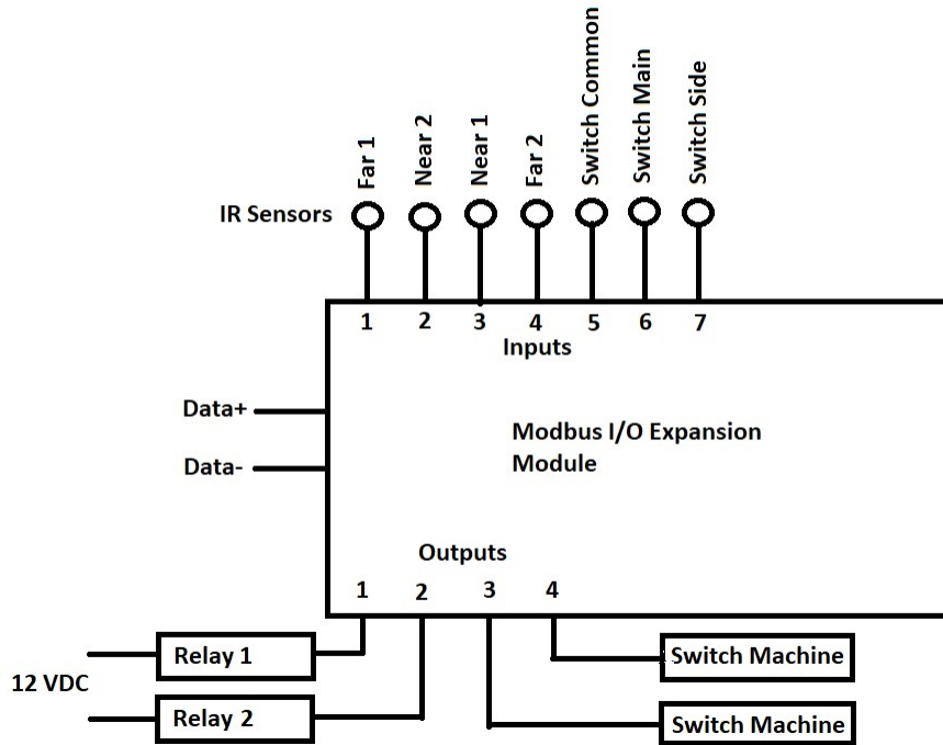
Fig. 5. Modbus I/O Expansion Module
