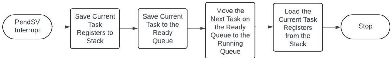
Fig. 8. PendSV Routine
