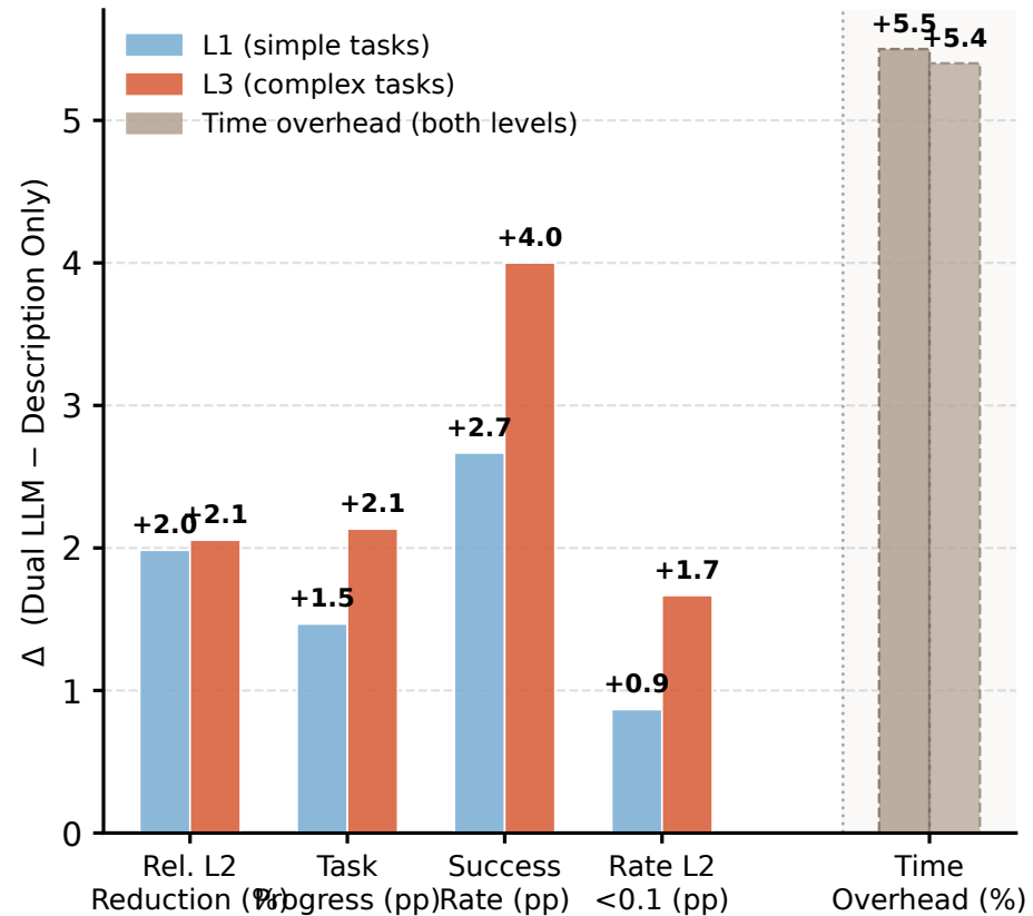
DreamZero / DROID
