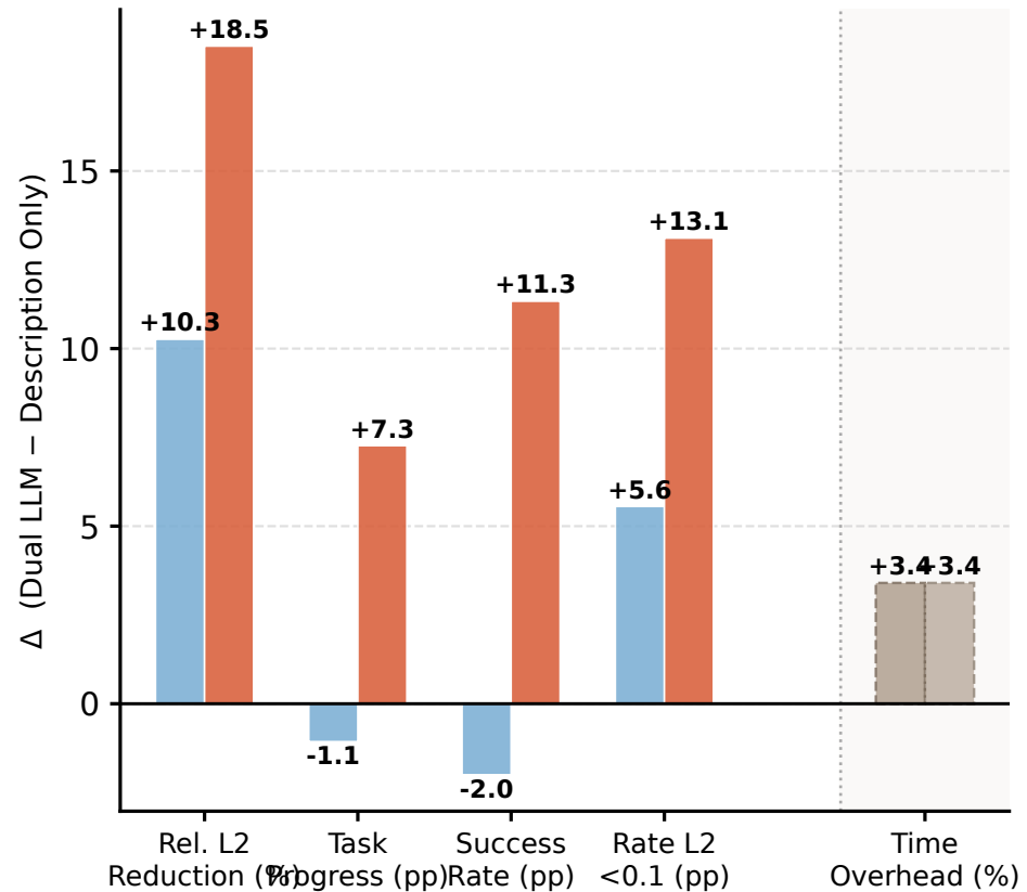
DreamZero / AgiBot
