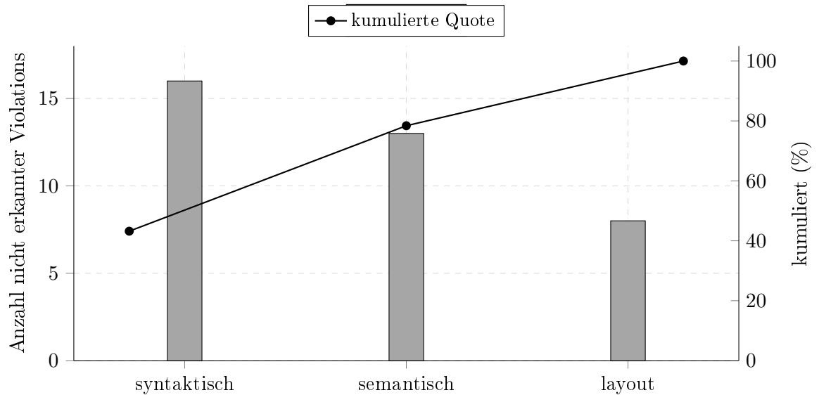
Abb. 16: Pareto-Auswertung der nicht konsistent erkannten Violations in test-100 (qwen3:32b). 78,4% der Ausfälle liegen bereits in den ersten zwei Kategorien (syntaktisch + semantisch). 237
