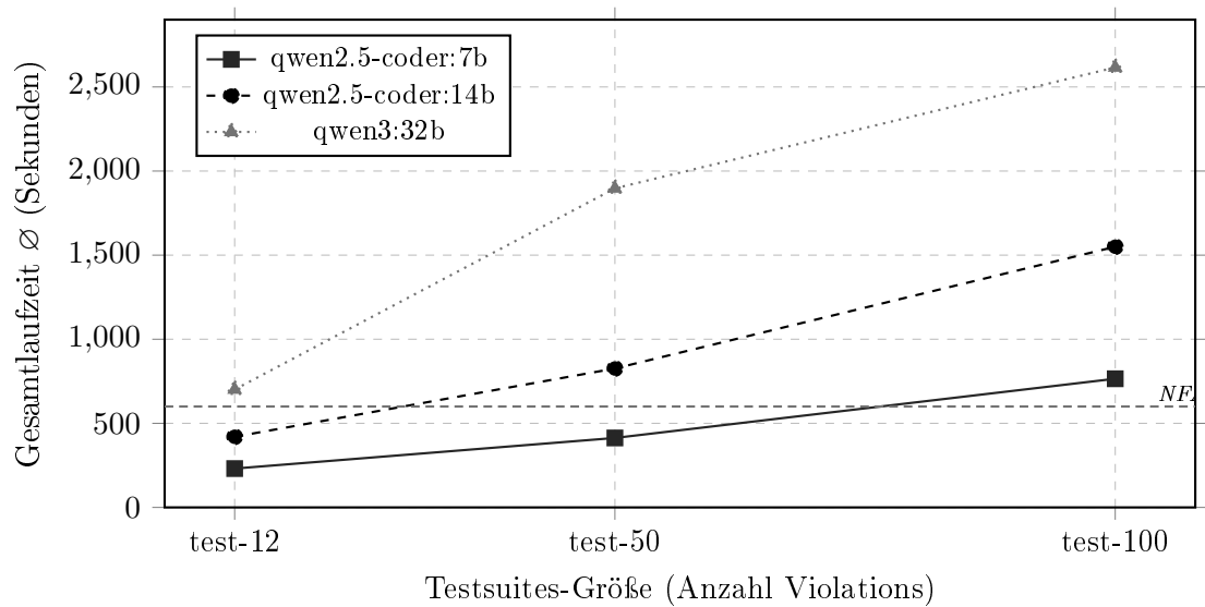
Abb. 26: Mittlere Gesamtlaufzeit in Sekunden je Modell und Testsuite. Die NFA-02-Grenzlinie markiert 600 s (10 Minuten). Datenbasis: Tabellen 32, 46, 59. 247
