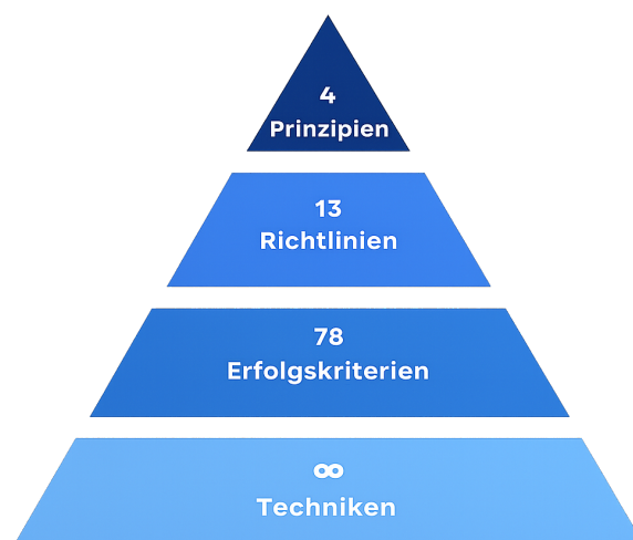
Abb. 1: WCAG-Schichtenmodell 62
