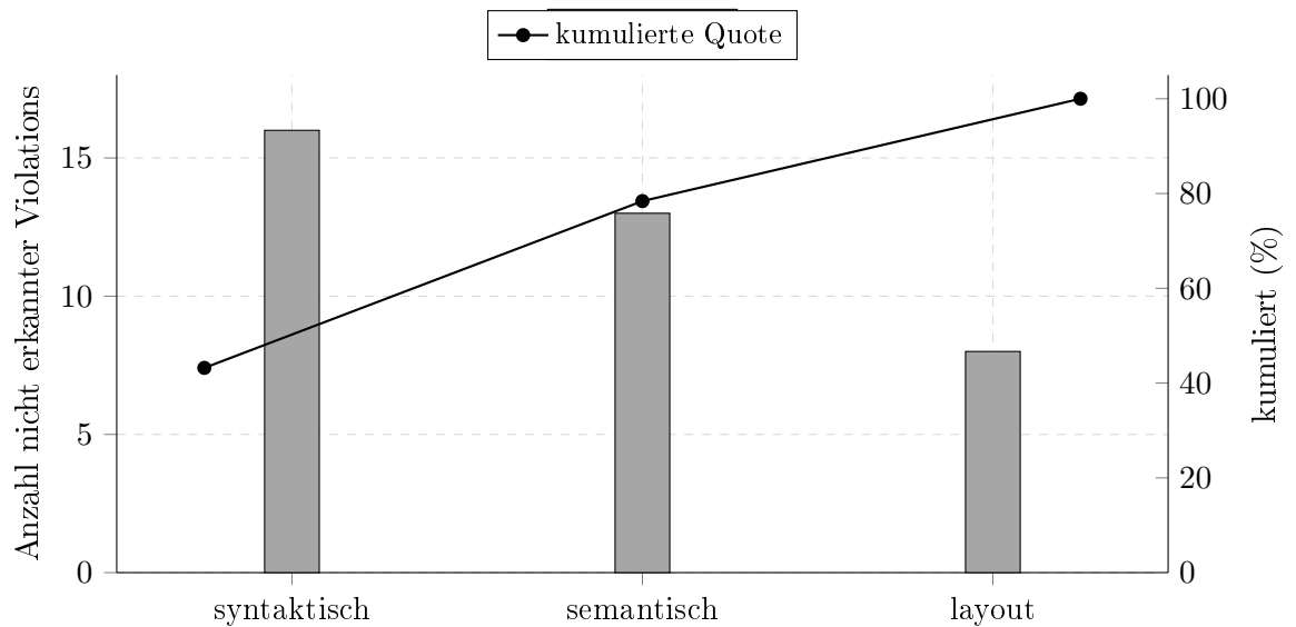
Abb. 15: Pareto-Auswertung der nicht konsistent erkannten Violations in test-100 (qwen3:32b). 78,4% der Ausfälle liegen bereits in den ersten zwei Kategorien (syntaktisch + semantisch). 245
