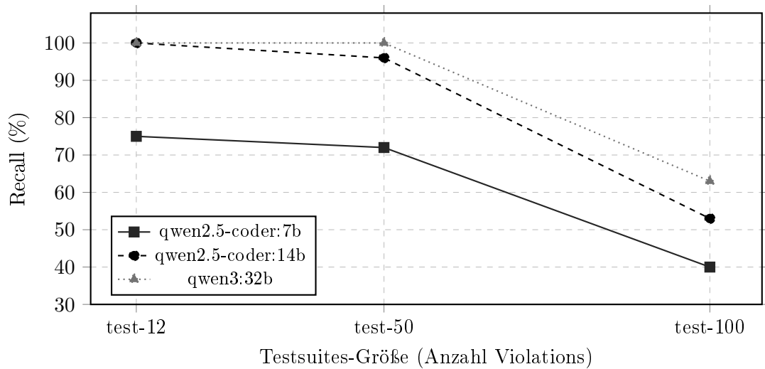
Abb. 24: Recall in Prozent je Modell über alle drei Testsuites (Konsistenzschwelle > 5/10 Runs). Der Knick zwischen test-50 und test-100 ist bei allen Modellen sichtbar. Datenbasis: Tabellen 31, 45, 58. 254
