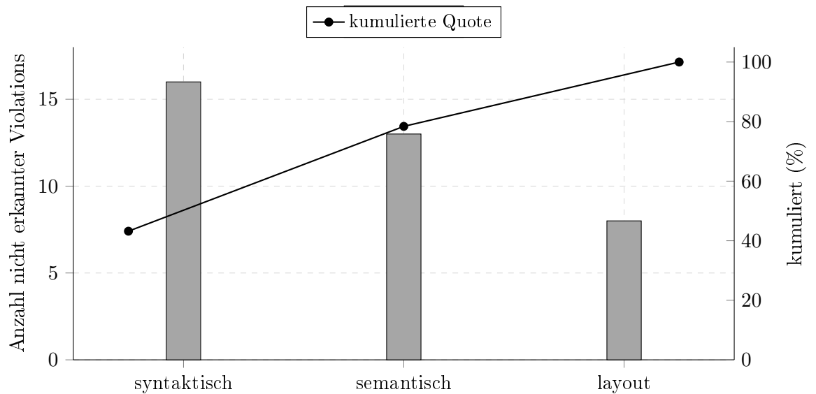
Abb. 16: Pareto-Auswertung der nicht konsistent erkannten Violations in test-100 (qwen3:32b). 78,4% der Ausfälle liegen bereits in den ersten zwei Kategorien (syntaktisch + semantisch). 241
