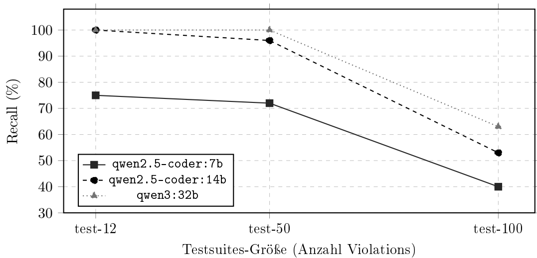
Abb. 24: Recall in Prozent je Modell über alle drei Testsuites (Konsistenzschwelle > 5/10 Runs). Der Knick zwischen test-50 und test-100 ist bei allen Modellen sichtbar. Datenbasis: Tabellen 28, 44, 58.
