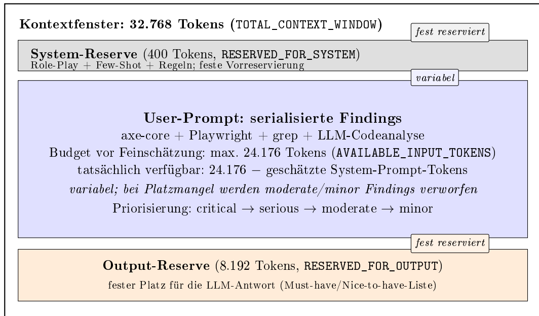
Abb. 8: Aufteilung des Kontextfensters (32.768 Tokens) gemäß Implementierung in src/prompt.ts : feste Reserven für System (400) und Output (8.192), variabler Bereich für serialisierte Findings mit Schweregrad-basierter Kürzung bei Budget-überschreitung. Die Abbildung zeigt ausschließlich Stufe 2 (Priorisierung); Stufe 1 (LLM-Detektor) besitzt ein separates, chunkweises num_predict -Budget (Default 640, Benchmark 2048). Vgl. Abschnitt 6.2.
