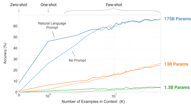
Abb. 5: Zero-Shot und Few-Shot Prompting im Vergleich 131
