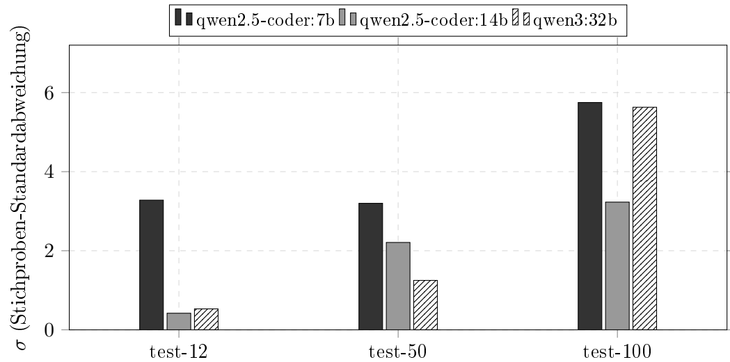
Abb. 27: Stichproben-Standardabweichung \sigma der LLM-Detektor-Findings je Modell und Testsuite ( n = 10 Runs). Niedrigere Werte bedeuten höhere Run-zu-Run-Konsistenz. Datenbasis: Tabellen 36, 50, 63. 260
