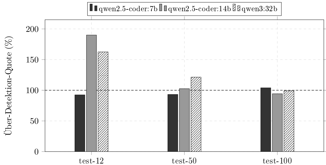
Abb. 28: Verhältnis der LLM-Detektor-Findings zur Ground Truth in Prozent. Werte über 100 % = Über-Detektion; darunter = Unter-Detektion. Die hervorgehobene Gitterlinie markiert die 100-%-Schwelle (exakte Übereinstimmung mit der Ground Truth). Datenbasis: Tabellen 35, 49, 62. 261
