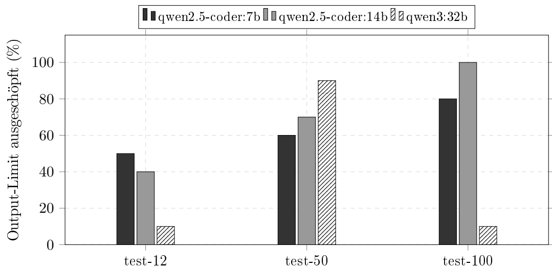
Abb. 29: Anteil der Runs mit ausgeschöpftem Output-Token-Limit je Modell ( n = 10 ). Das num_predict -Budget wurde skaliert: test-12: 6 144, test-50: 8 192, test-100: 12 288 Tokens. Der Rückgang bei qwen3:32b von 90 % (test-50) auf 10 % (test-100) erklärt sich durch dessen kompaktere JSON-Ausgabestruktur. Datenbasis: Tabellen 32, 46, 59. 262
