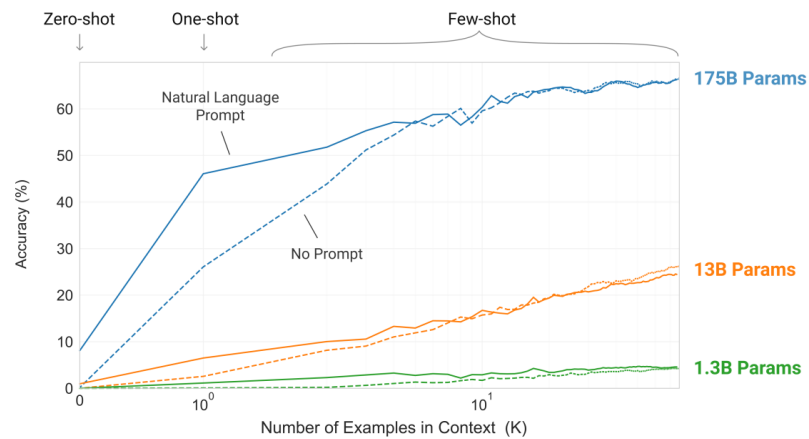
Abb. 5: Zero-Shot und Few-Shot Prompting im Vergleich 146
