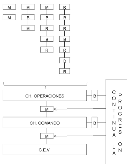
FASE DE OP's. AEROTACTICAS FLUJOGRAMA DE PROCEDIMIENTOS PARA SEPARACIÓN DE VUELOS
