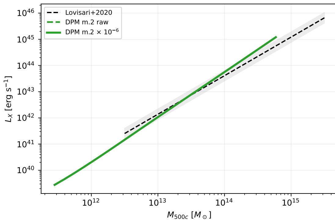
L_X - M : unit correction
