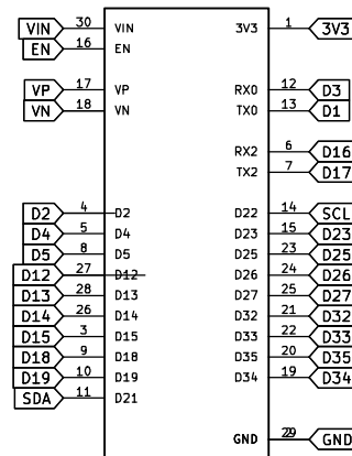
U1 ESP32-DEVKIT-V1
