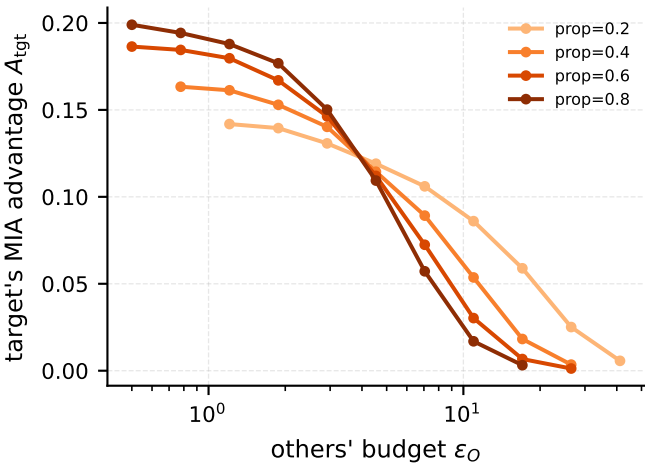
target \varepsilon_T = 4
