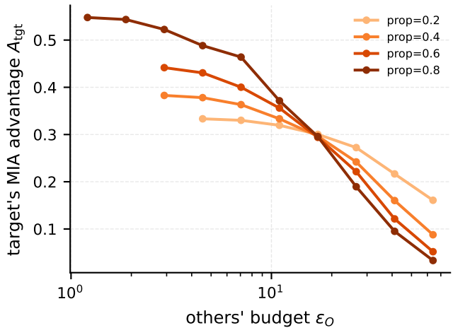
target \varepsilon_T = 16
