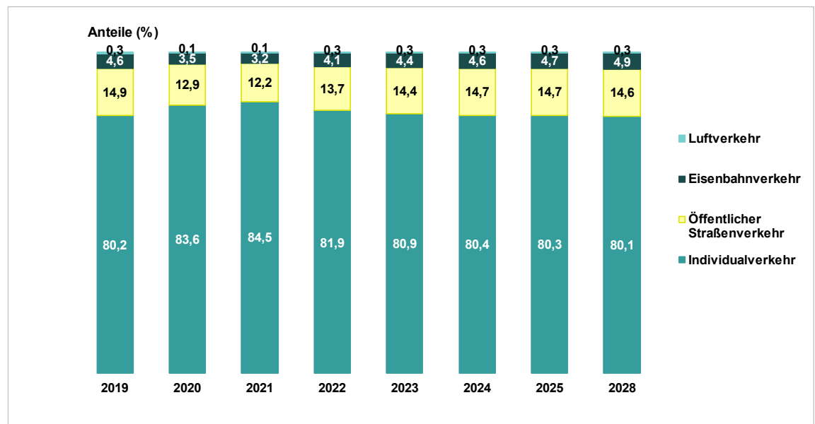
Abbildung P - 1: Modal Split des Personenverkehrsaufkommens
