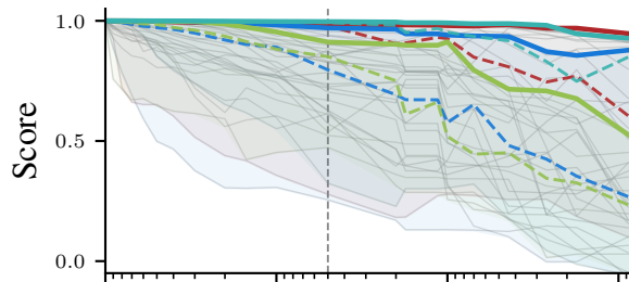
tRSA
