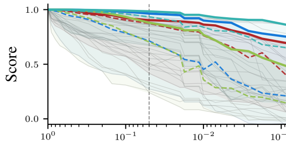
tRSA
