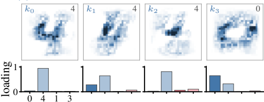
(d) even circuit — L_1 factors below L_2 k_0
